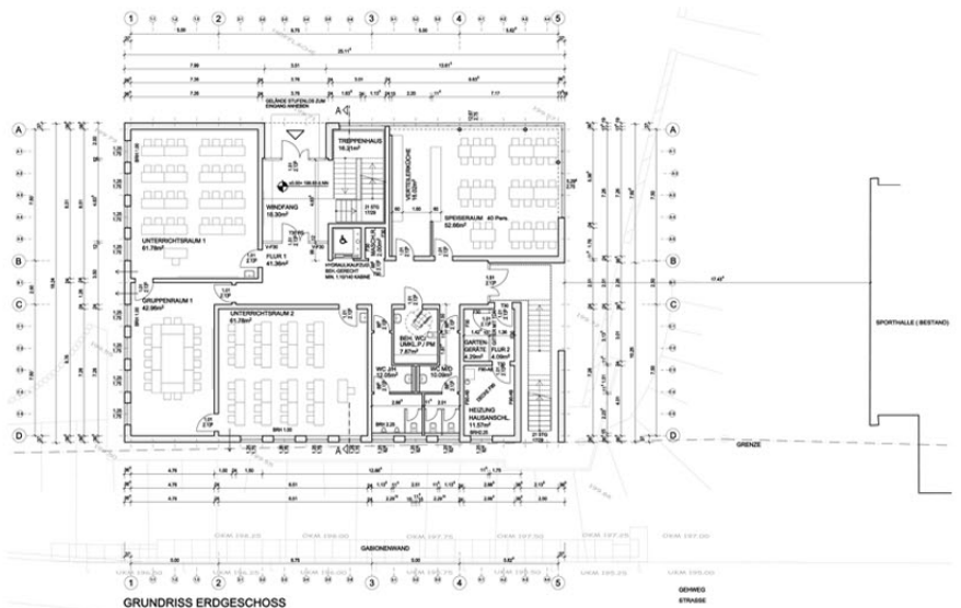
Grundriss EG
