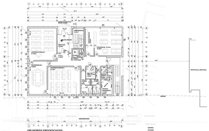
Grundriss EG
